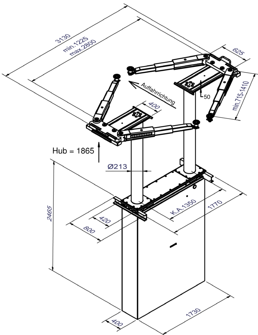
Przesuwna głowica
