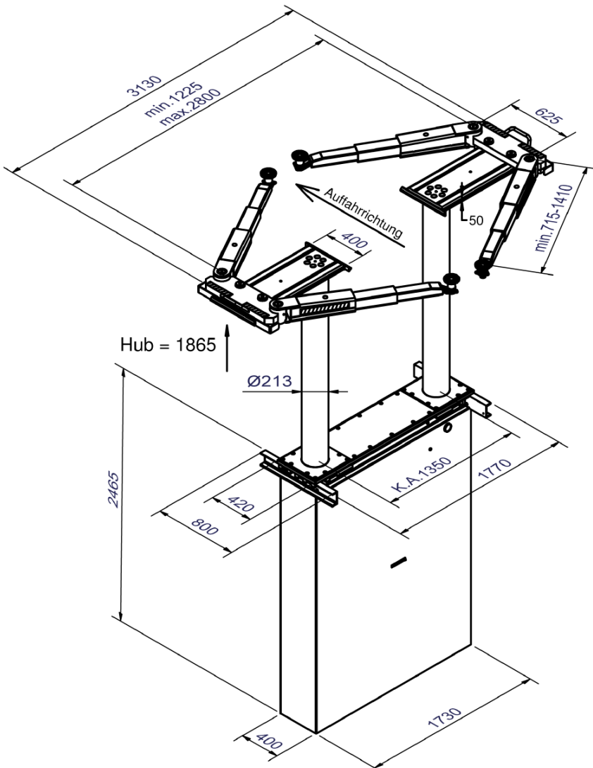
Przesuwna głowica
