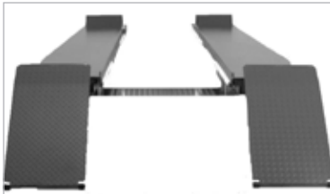
Profilift 2.40 F 460 VAS 5248
